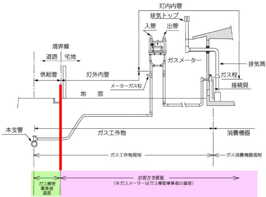
図 3.1.9 導管の区分
